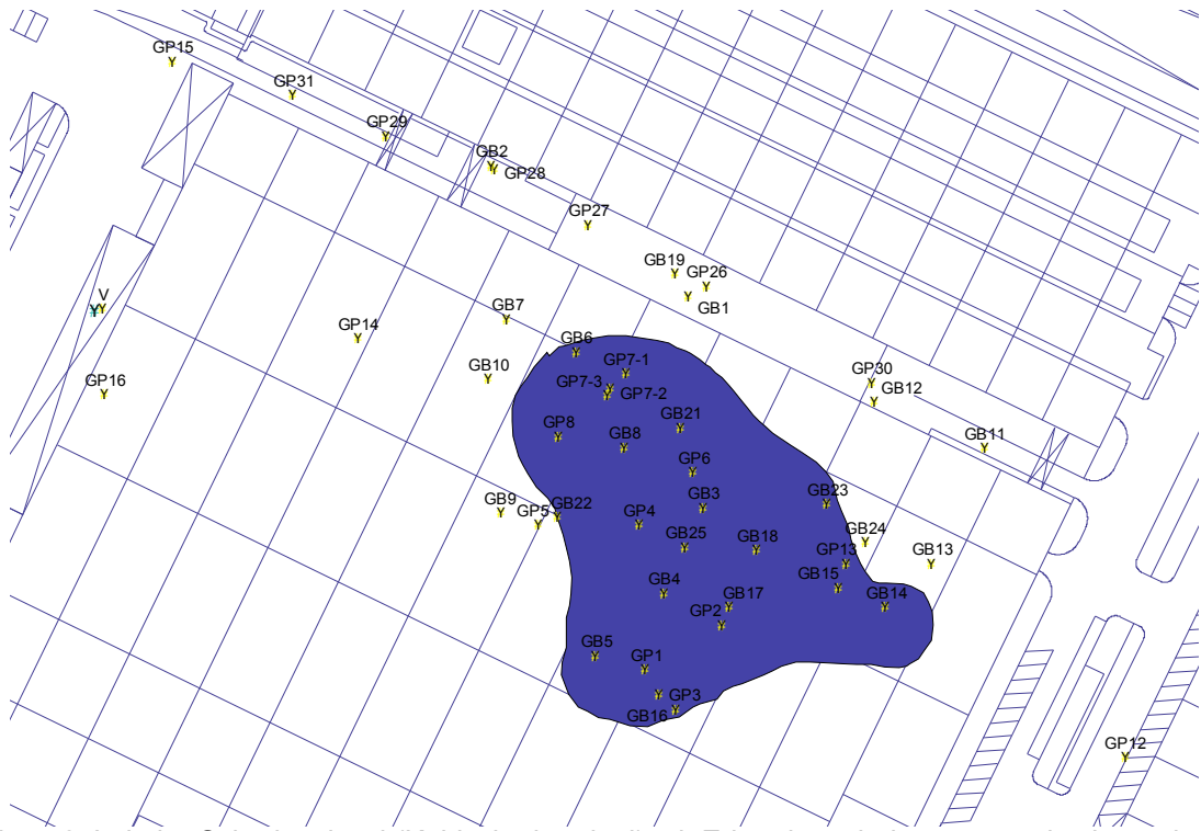
Abbildung 2: Lokaler Schadensherd (Kühlschmiermittel) mit Erkundungsbohrungen und schematischer Ausdehnung der freien bzw. residualen Phase.
